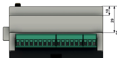
Rysunki i wymiary (wszystkie wymiary w milimetrach)
