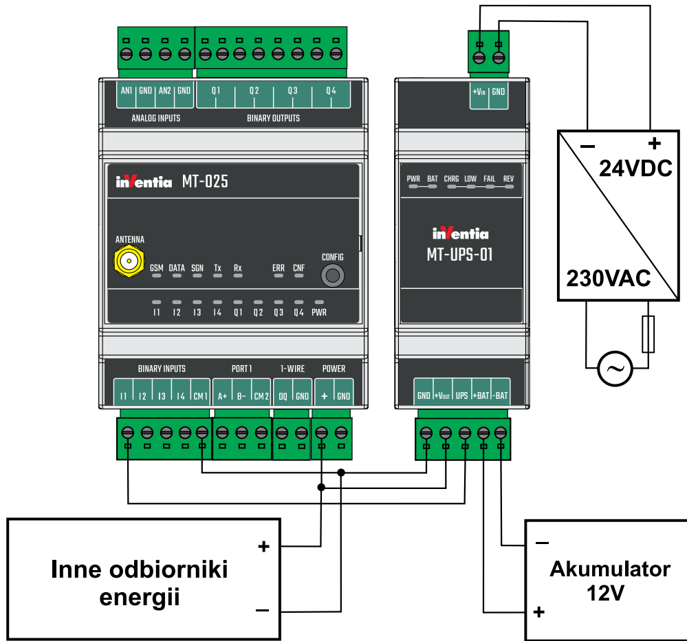
Przykład podłączenia modułu MT-UPS-1 do modułu telemetrycznego MT-025
